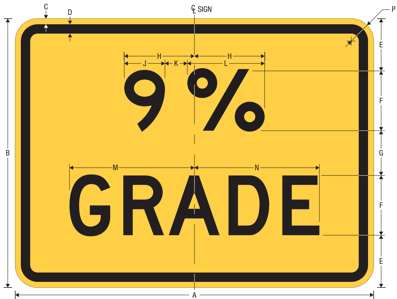
W7-3P XX% GRADE (PLAQUE)
