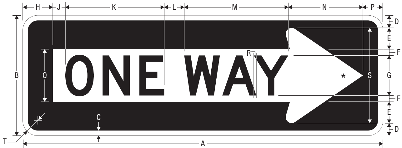
R6-1R ONE WAY
