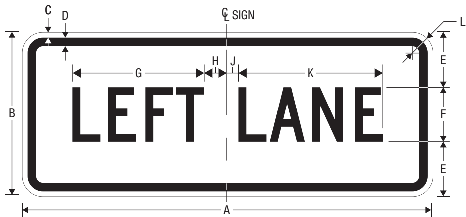
R3-5bP LEFT LANE (PLAQUE)
