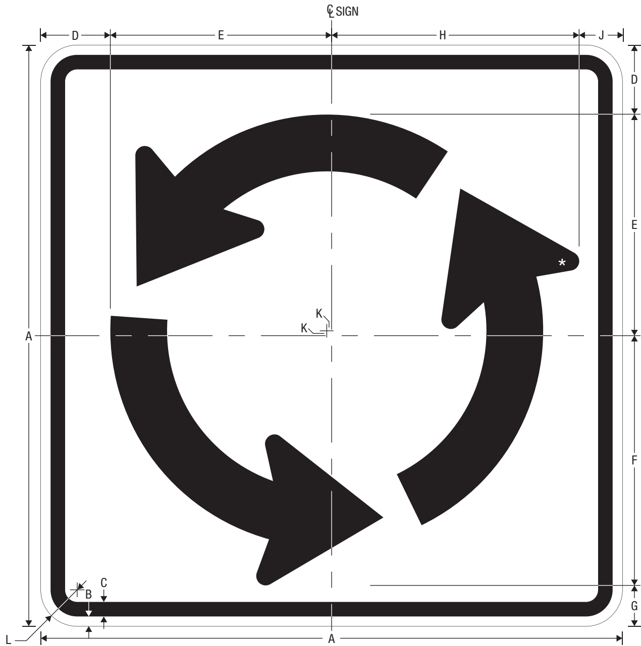
R6-5P ROUNABOUT CIRCULATION (PLAQUE)
