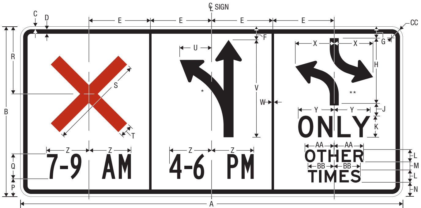
R3-9e REVERSIBLE LANE CONTROL (OVERHEAD)
