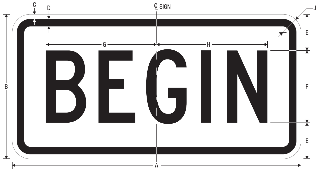
R3-9cP BEGIN (PLAQUE)
